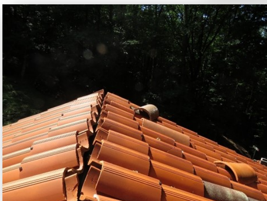
Tetto Capanna Bonardi Mazzoleni prima e dopo intervento
