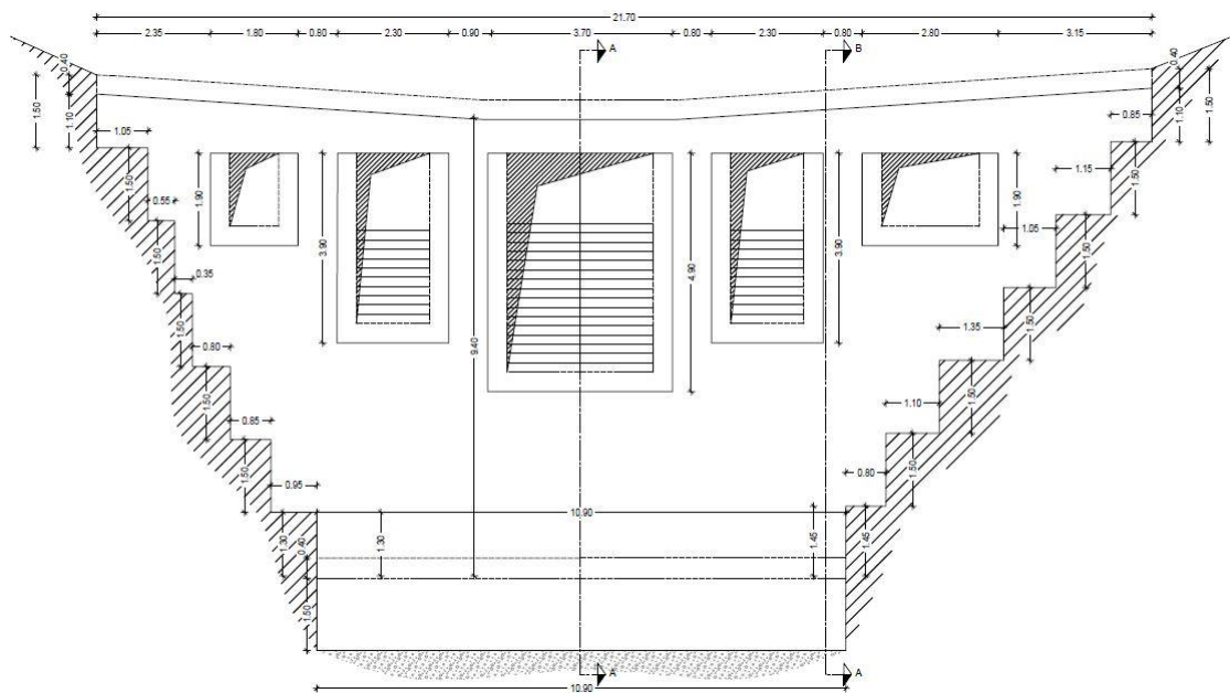
Prospetto della nuova briglia
