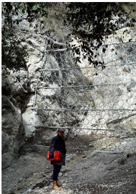
Figura 3 - Barriera di contenimento n. 1 installata in alveo appena a monte della strada di accesso al villaggio vacanze "La Limonaia" – vista da valle
