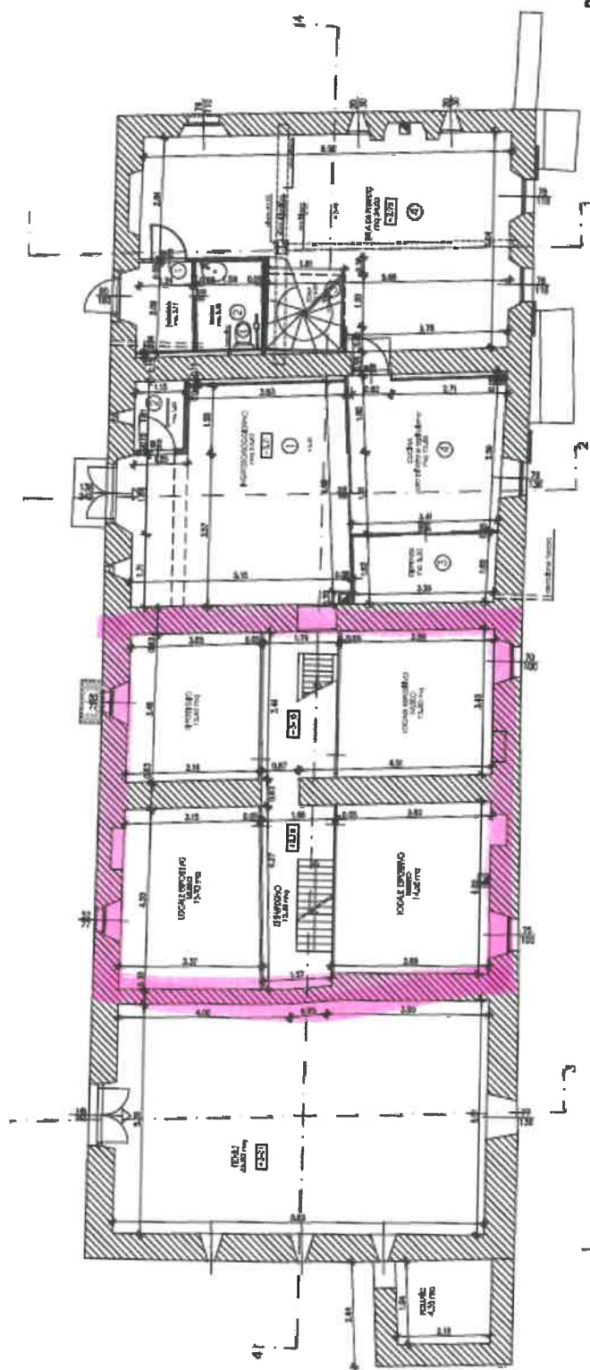
Piano Primo
