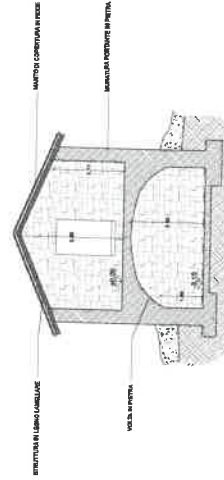
Sezione A-A
